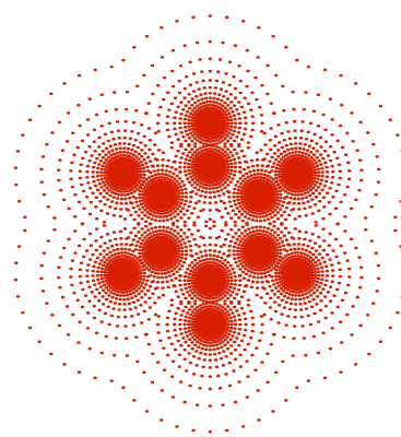
(d) \text{C}_6\text{H}_6
