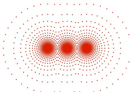
(b) \text{CO}_2
