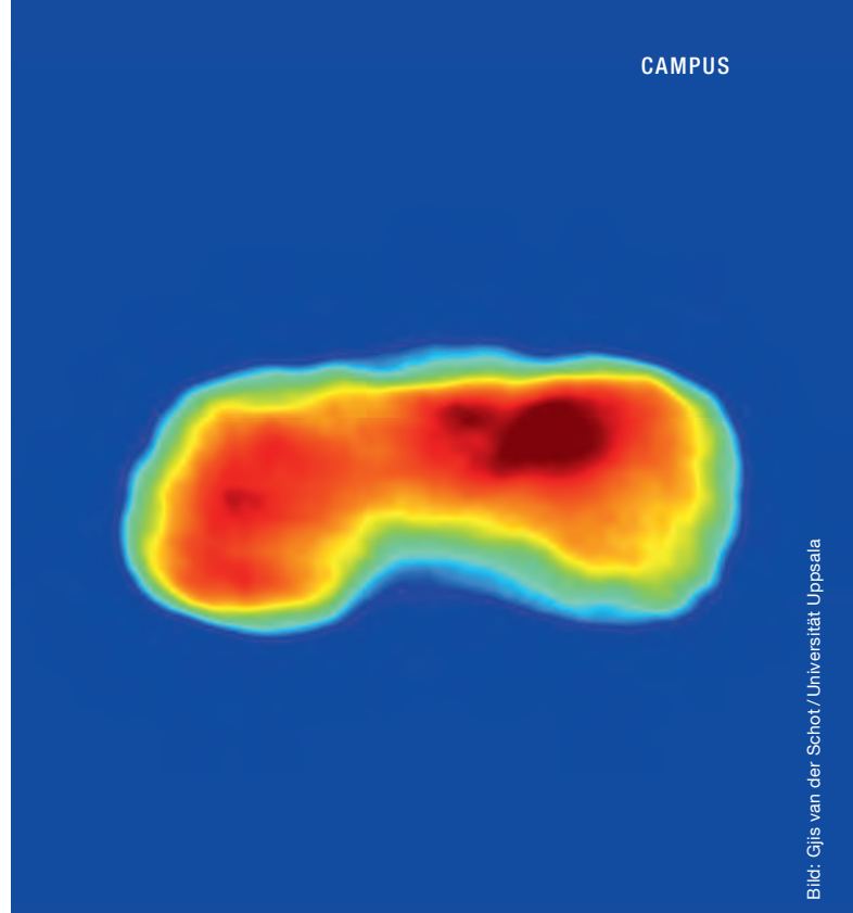
Rekonstruktion eines Cyanobakteriums aus dem Röntgenstreubild
