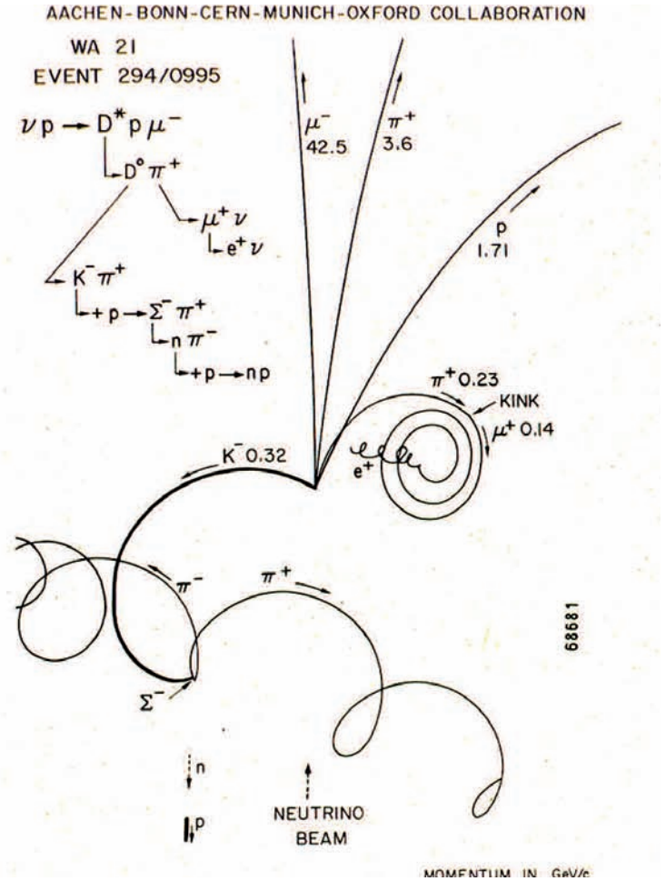
Abb. 9: Reaktion eines von unten kommenden (unsichtbaren) Neutrinos mit einem Proton ( p ). Hierbei entstehen ein negativ geladenes Myon ( \mu^- ), ein Proton und ein angeregtes Meson D^* . Letzteres zerfällt rasch in ein D^0 -Meson und ein \pi^+ -Meson ( \pi^+ ). (Foto: CERN)
