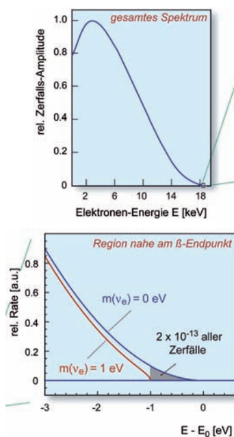
Das Energiespektrum von Elektronen aus dem Tritium-Betazerfall zeigt nahe am kinematischen Endpunkt eine charakteristische Modifikation in Abhängigkeit von der Neutrinomasse.
