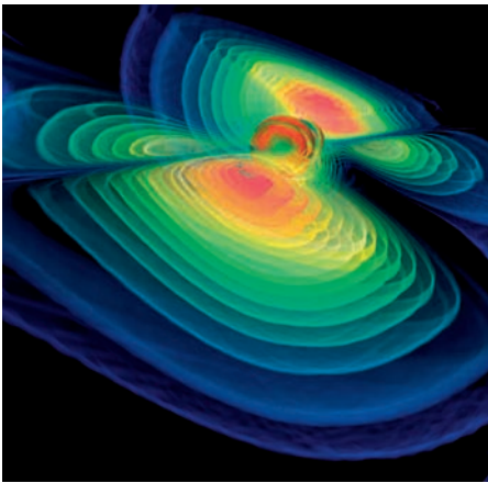
Computersimulation von zwei miteinander verschmelzenden Schwarzen Löchern. Die farbigen zwiebelartigen Strukturen zeigen die sich entfernenden Gravitationswellen. Die schalenförmigen scheinbaren Horizonte der Schwarzen Löcher im Mittelpunkt der Grafik sind dunkelrot gekennzeichnet (MPI für Gravitationsphysik und ZIB, W. Bengert mit Amira).
