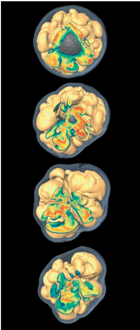
Dreidimensionale Computersimulation einer Supernova. Die Bilder zeigen die durch Neutrinos verursachte Konvektion um den entstehenden Neutronenstern. Wegen rechtechnischer Grenzen kann die Neutrinophysik in solchen Simulationen derzeit nur näherungsweise behandelt werden.
