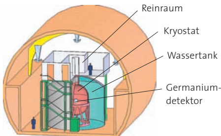
Schematischer Aufbau von GERDA. Die Germanium-detektoren werden über einen Reinraum in den Flüssigstickstofftank eingeführt. Ein vakuumisolierter Tank mit etwa vier Meter Durchmesser ist von einem Wassertank mit etwa zehn Meter Durchmesser eingeschlossen. Beide zusammen schirmen die Störstrahlung aus der Felswand ab. Der Wassertank und der darin befindliche Tscherenkow-Detektor dient darüber hinaus zum Nachweis von kosmischen Myonen, die Störsignale verursachen können.
