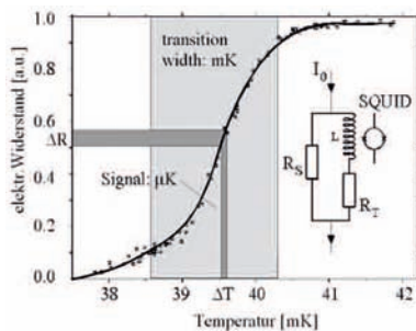
Unterhalb einer kritischen Temperatur verliert der supra-leitende Film sehr schnell vollständig seinen elektrischen Widerstand. Wird der Film bei seiner kritischen Temperatur stabilisiert, führen kleine Temperaturschwankungen zu großen und damit messbaren Schwankungen im elektrischen Widerstand.
