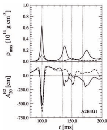
Verlauf von Materiedichte und Gravitationswellenamplitude beim Gravitationskollaps eines rotierenden Sterns (gestrichelt: Newtonsche Beschreibung der Bewegung des Sterns, durchgezogen: allgemein-relativistische Beschreibung der Bewegung des Sterns) (MPA, Dimmelfmeier).
