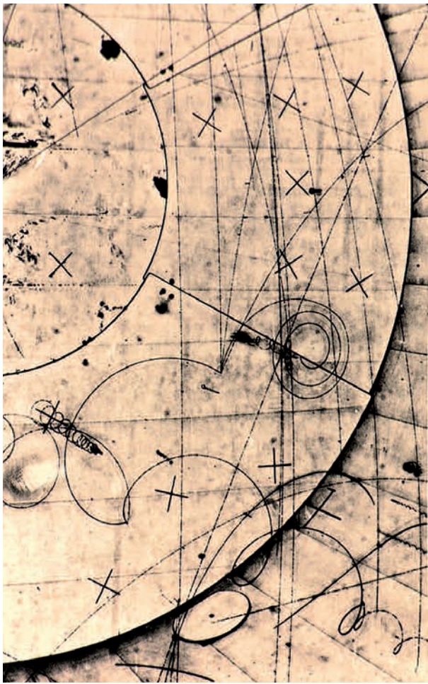
Abb. 9: Reaktion eines von unten kommenden (unsichtbaren) Neutrinos mit einem Proton ( p ). Hierbei entstehen ein negativ geladenes Myon ( \mu^- ), ein Proton und ein angeregtes Meson D^* . Letzteres zerfällt rasch in ein D^0 -Meson und ein \pi^+ -Meson ( \pi^+ ). (Foto: CERN)
