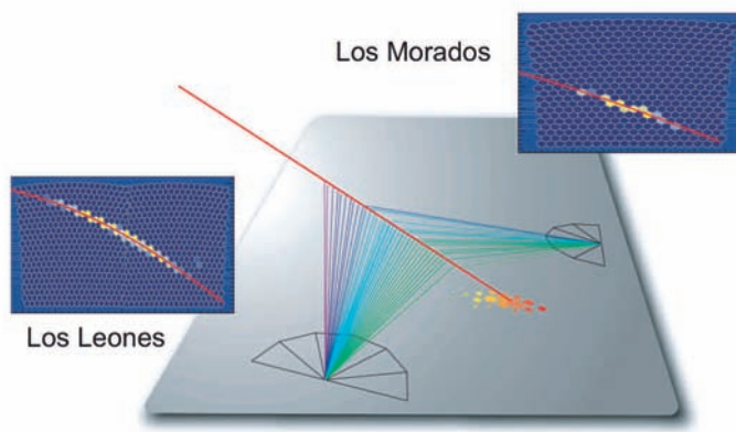
Darstellung eines Luftschauers, der von den Fluoreszenzteleskopen im Stereomodus beobachtet wurde und dessen Teilchen in 17 Tanks des Oberflächenfelds nachgewiesen wurden (Stereo-Hybrid-Ereignis). Die Schauerachse ist als rote Linie zusammen mit der entsprechenden Projektion auf die von den Teleskopkameras aufgenommenen Bilder dargestellt. Die rekonstruierte Energie des Schauers beträgt 2 \cdot 10^{19} eV.
