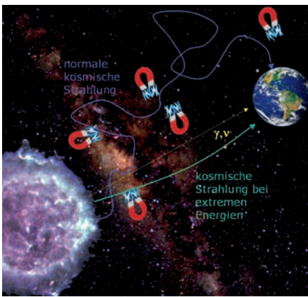
Abb. 19: Elektrisch geladene Teilchen werden in den interstellaren Magnetfeldern unseres Milchstraßensystems abgelenkt. Nur Teilchen mit den höchsten Energien sowie die neutralen Neutrinos fliegen auf geradlinigen Bahnen.
