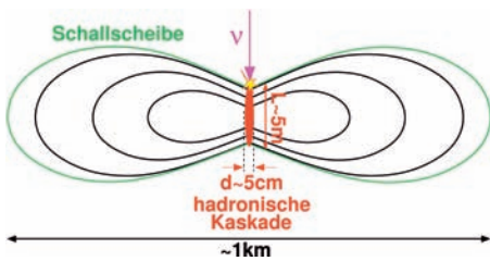
Ein Neutrino erzeugt nach einer Wechselwirkung in Wasser oder Eis einen Teilchenschauer, der senkrecht dazu Schall in Form einer Scheibe abstrahlt.
