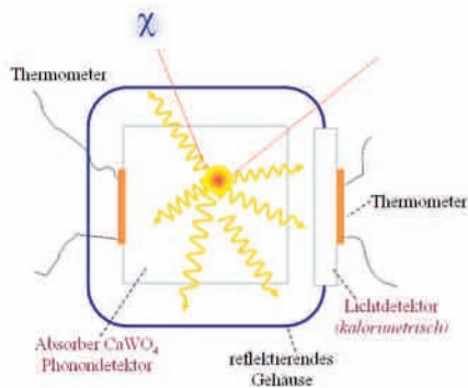
Das Nachweisprinzip der CRESST-Detektoren beruht auf zwei Effekten: Einer Temperaturerhöhung und gleichzeitig erzeugtem Szintillationslicht.
