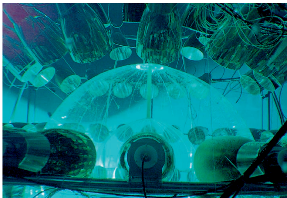
Der Prototypdetektor CTF, bestehend aus vier Tonnen Szintillator in einem Nylonballon mit zwei Meter Durchmesser, umgeben von hundert Photosensoren, die das Szintillationslicht registrieren.
