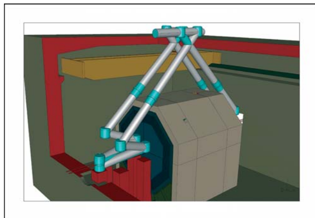
Abbildung 78: Integration des Laser-Resonators in den Detektor.
